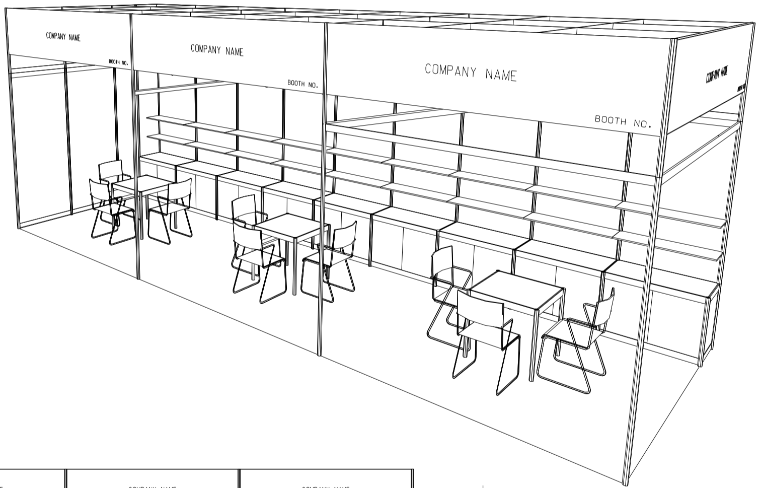
PERSPECTIVE 9M(W) X 3M(D) X 3.5M(H)
